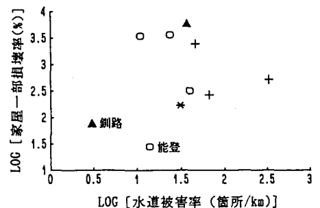
図6 地中管路被害率と家屋一部損壊率との関係
