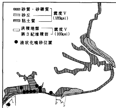
図2 珠州市の地盤種別と地震時震度、液状化状況
