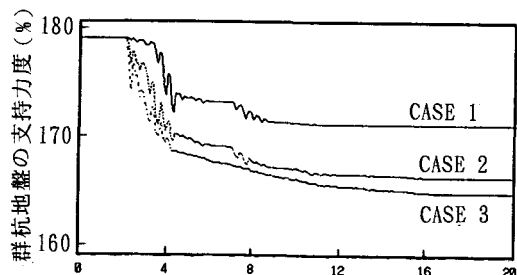
図-6 群杭地盤の支持力度 (s)
