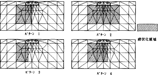
図-2 液状化領域図
