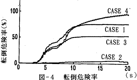
図-4 転倒危険率
