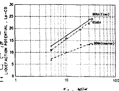
図3 側圧と Lp_{-CD}
