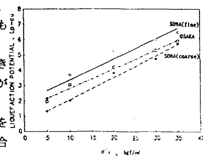
図4 側圧と Lp_{-CU}
