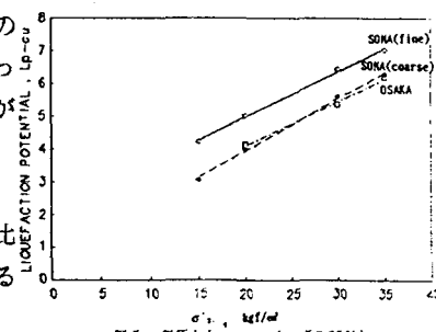
図5 側圧と Lp_{-CU} (ひずみ25%)
