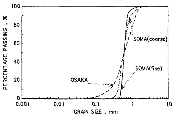
図.1 粒度曲線
