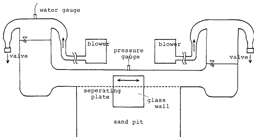
図-1 実験装置
