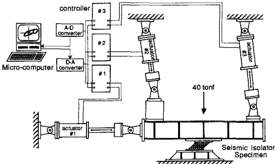
図-1 実験システムの全体図
