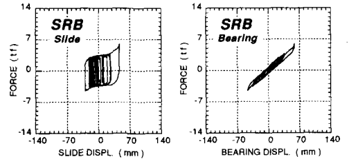
図-3 SRBの履歴曲線の分離
