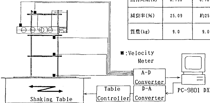
図1 実験システムのブロックダイアグラム
