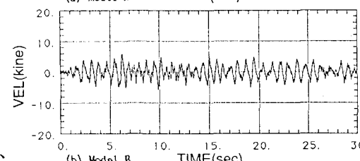
図4 フィルタードホワイトノイズ波入力時3層速度時刻歴
