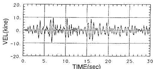
図6 3層に対するTMDの相対速度時刻歴
