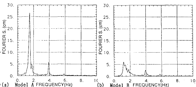
図5 フィルタードホワイトノイズ波入力時3層速度フーリエスペクトル
