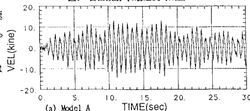
図3 自由振動時3層速度時刻歴
