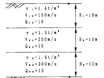
図-5 基盤上の3層地盤モデル
