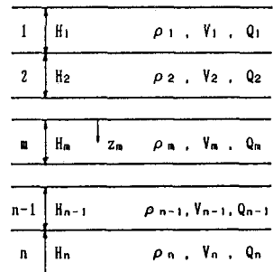
図-1 水平成層地盤モデル
