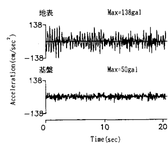
図-3 加速度波形
