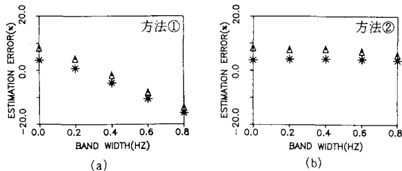
図-4 Q値の推定誤差(ノイズ5%*, 10%△)
