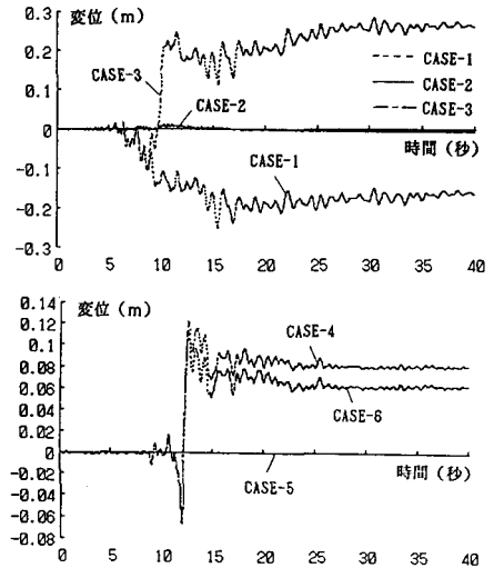
図3 A点の水平方向応答変位
