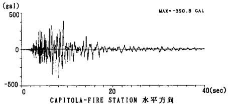
図2 入力地震波
