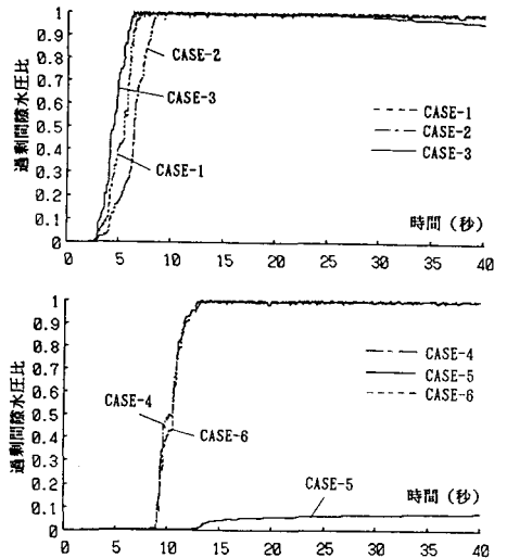
図4 A点の過剰間隙水圧比
