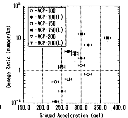
図-6 水道石棉管の被害率
