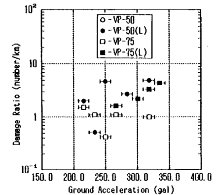
図-7 水道塩化ビニール管の被害率
