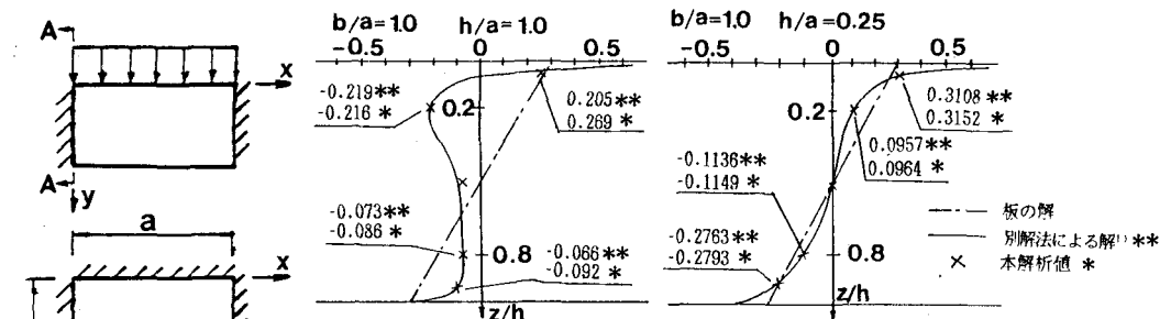
図-6 \sigma_x の応力分布 ( qa^2/h^2 ) A-A断面
