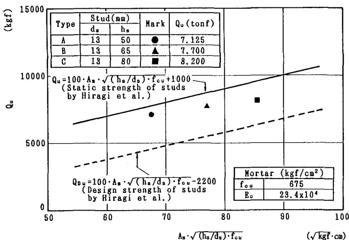
図-2 各タイプの破壊荷重の比較
