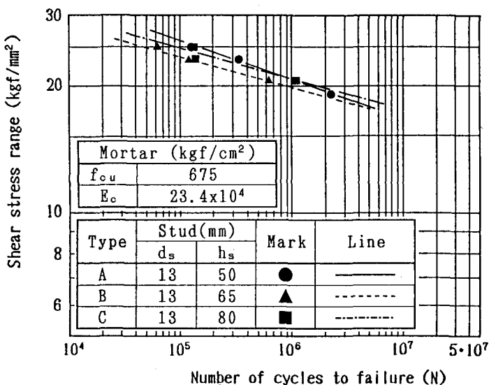
図-3 各タイプのS-N関係の比較
