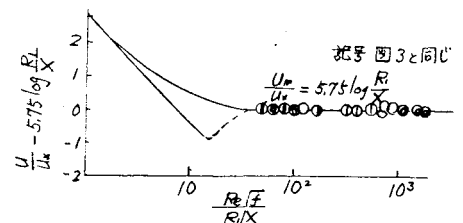
図5 X の普遍的性質
