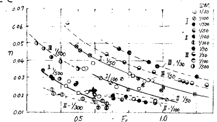
図3 木津川模型の粗度係数 n
