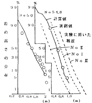
図2 式(1), 式(6)による計算と実測との比較及び実験に用いた石の大きさ
