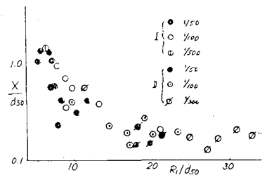
図4 木津川の粗度要素 X
