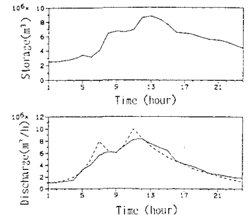
図5 分散を導入したときの制御結果
