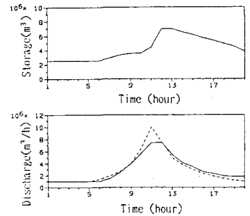
図3 ファジィ制御による結果
