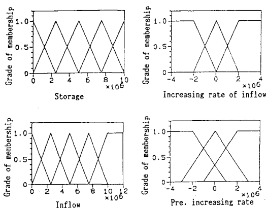
図1 前件部のメンバーシップ関数
