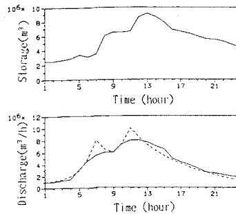
図4 平均値のみの場合の制御結果
