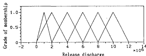
図2 後件部のメンバーシップ関数
