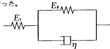
図-1 3要素モデル
