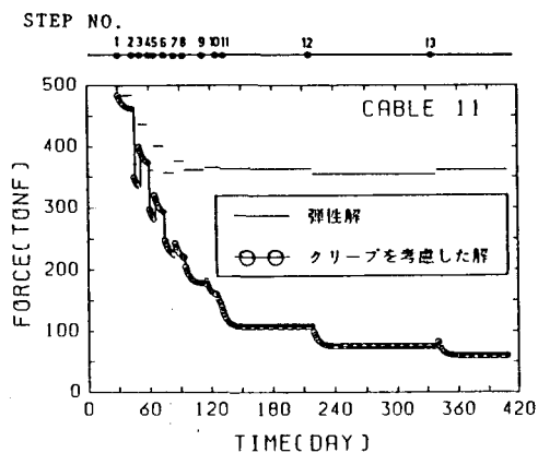
図-5 ケーブル11の張力の経時挙動
