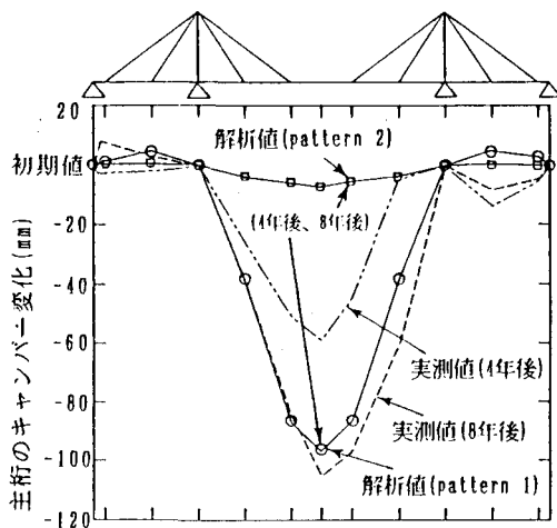
図-6 実測値と解析値の比較
