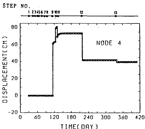
図-4 節点4の変位の経時挙動
