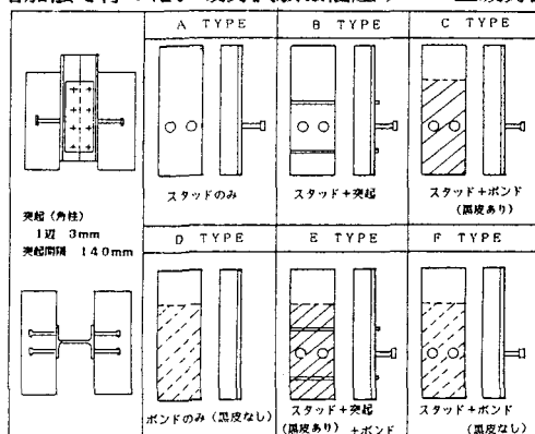
図-1 押抜き供試体の種類
