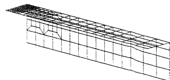
図-4 有限要素法解析の要素分割
