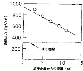
図-1 横桁上フランジの応力分布
