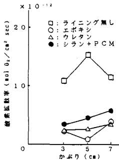
図-3 ライニング仕様が酸素拡散率に与える影響
