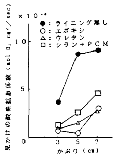
図-7 ライニング仕様が見かけの酸素拡散係数に与える影響
