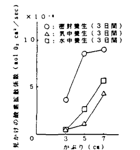
図-8 養生条件が見かけの酸素拡散係数に与える影響
