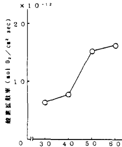
図-5 水セメント比が酸素拡散率に与える影響
