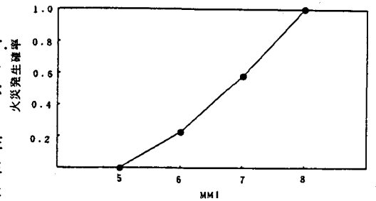
図3 火災発生率とMMI震度階の関係
