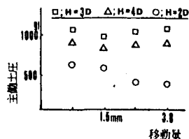
図-3 壁板の移動と主働土圧
