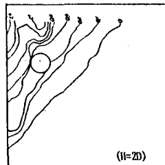
図-5 Y成分の等移動量曲線
