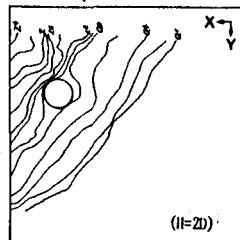
図-4 X成分の等移動量曲線
