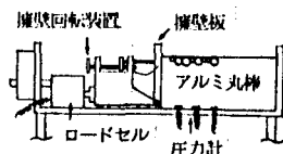
図-1 すべり面発生装置
