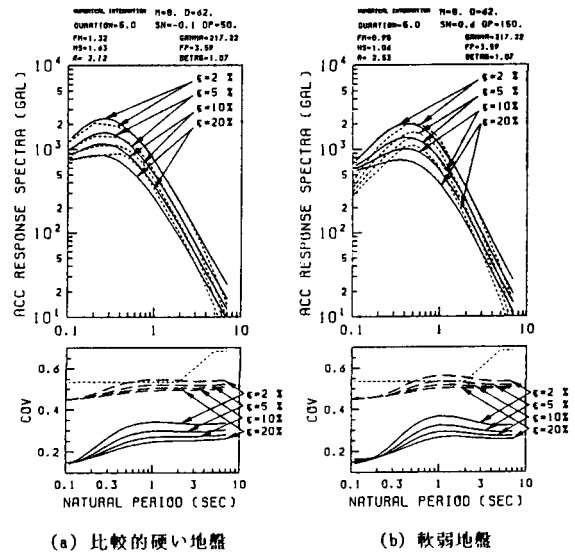
図2 地表面における応答スペクトル (M=8, Δ=62)
