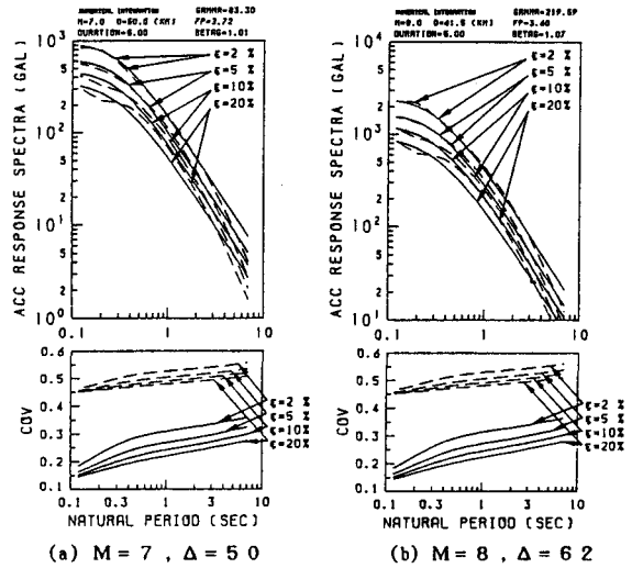
図1 工学的基盤面における応答スペクトル
