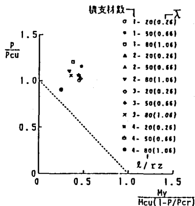
図-4 立体解析モデル 耐荷力相関図 (A-Type) (有効座屈長 面内 0, 面外 l )
