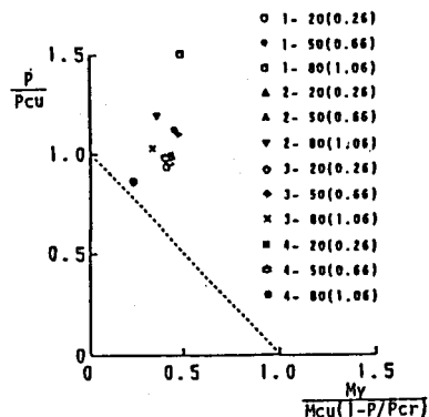
図-5 立体解析モデル 耐荷力相関図 (B-Type) (有効座屈長 面内 0, 面外 l )
