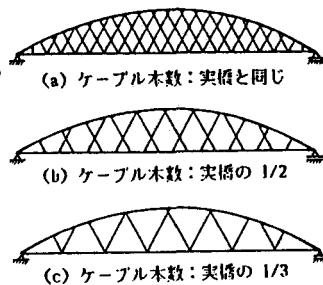
図-1 平面解析モデル
