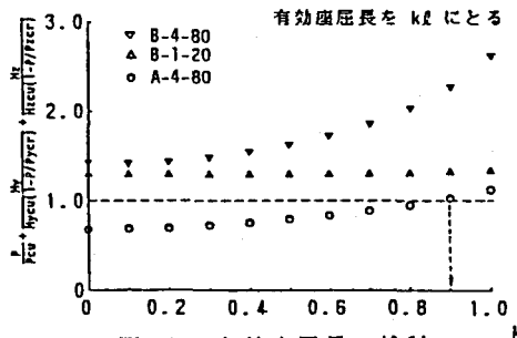
図-6 有効座屈長の検討
