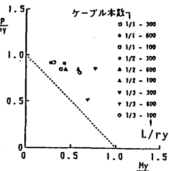
図-3 平面解析モデル 耐荷力相関図 (有効座屈長 面内 0, 面外 0)
