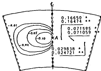
換算せん断力 ( V_\theta ) の影響面 (A点)
