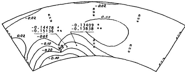
曲げモーメント ( M_\theta ) の影響面 (B点)
