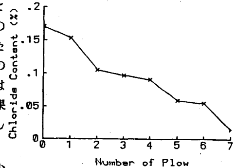
図-3 各スキ通過後の塩化物濃度
