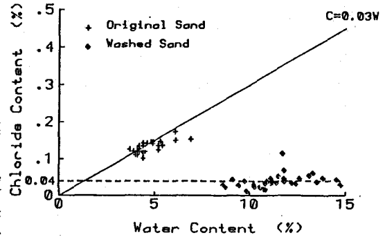
図-2 含水率と塩化物濃度の関係
