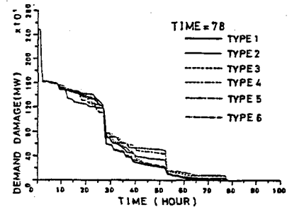
図6. 復旧戦略の相違による復旧過程
