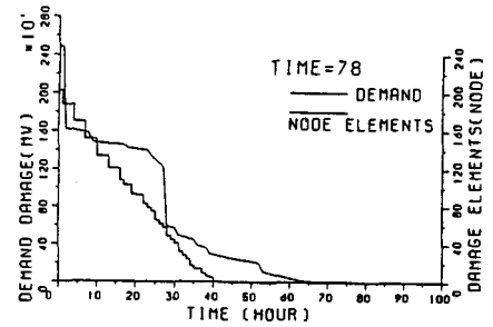
図4. 停電量と変電所の被災要素の復旧過程
