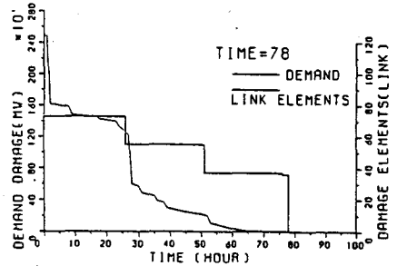
図5. 停電量と送電線変電所の被災要素の復旧過程
