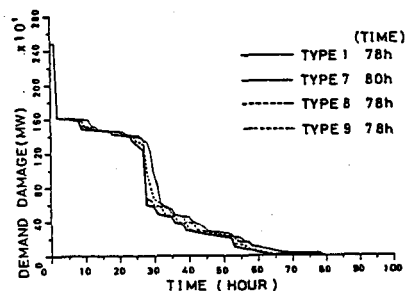
図7. 復旧人員の集合状況の相違による復旧過程
