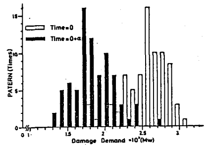
図1. 系統切替前、及び切替後の停電量
