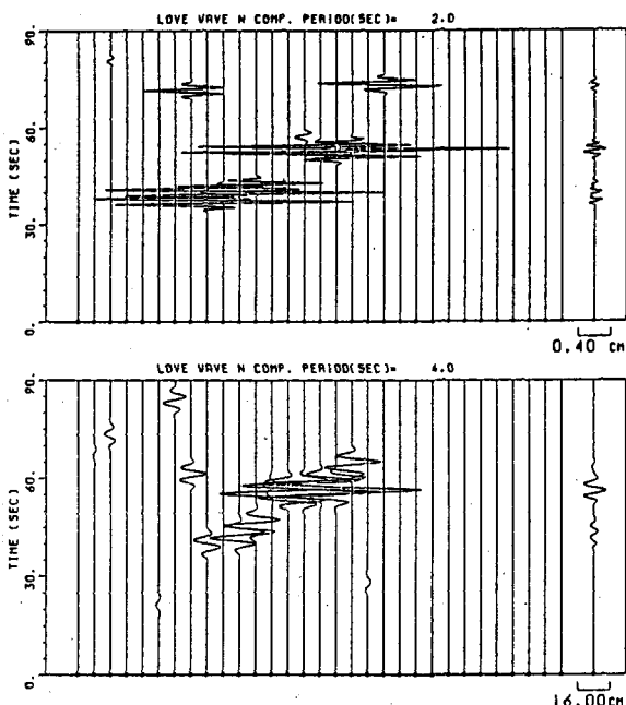
図6 合成波形図
