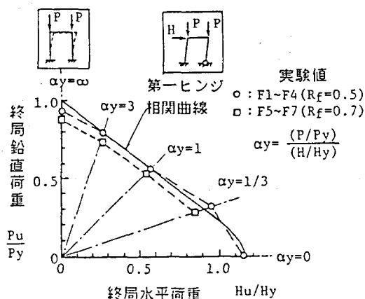
図-4 終局の鉛直荷重と水平荷重との相関関係
