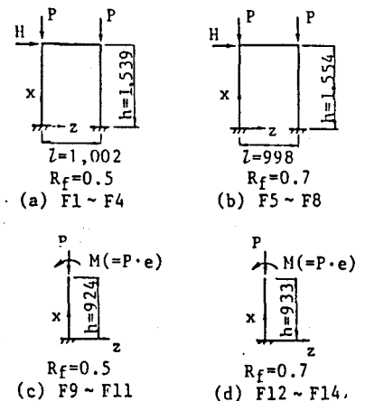
図-1 供試体の実測骨組寸法 (mm)
