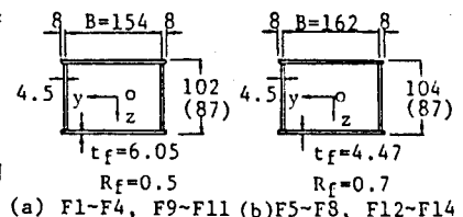
( ) 内は梁断面寸法 図-2 実測断面寸法 (mm)
