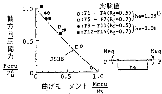
図-3 座屈強度の実験値とJSHBの耐荷力相関式との比較
