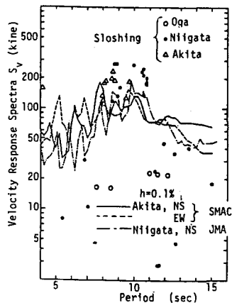
図5 JMA, SMACの S_v 値
