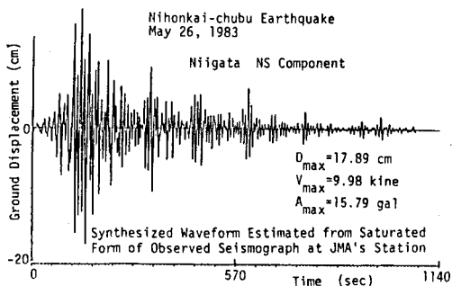
図7 修正・補正した新潟のJMA記録
