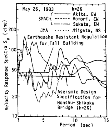
図6 各種設計基準との比較
