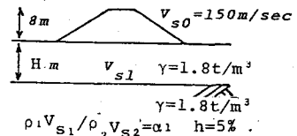
図-1 盛土地盤系モデル
