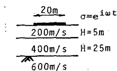
図-5(a) 地盤モデル
