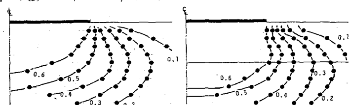
図-4(c) せん断応力分布 (5Hz)
