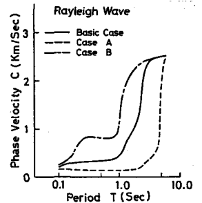
図2 第1中間層の \beta の変化による位相速度
