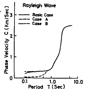
図1 地表の \beta の変化による位相速度
