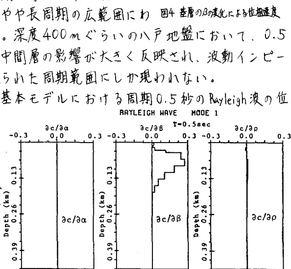
図5 基本モデルにおける各層の物理定数の位相速度に与える影響度
