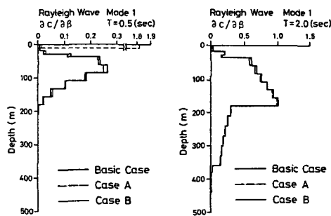
図6 地表層の \beta の変化による \partial c/\partial \beta
