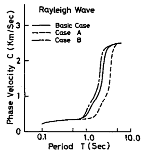
図3 第2中間層の \beta の変化による位相速度
