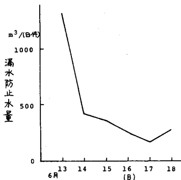
図-3 漏水防止水量の推定値の推移
