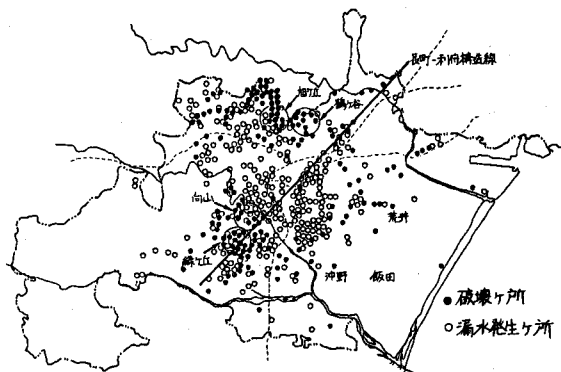
図-1 仙台市配水管被害ケ所分布図(宮城県沖地震)
