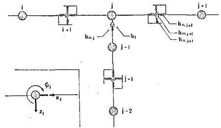
図-2 桁・橋脚の力要素と座標
