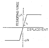
図-4 支承の弾塑性モデル
