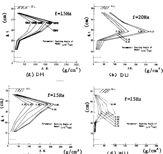
図3 振動土圧の鉛直分布
