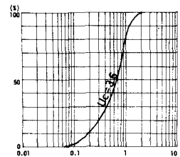
図2 粒径加積曲線
