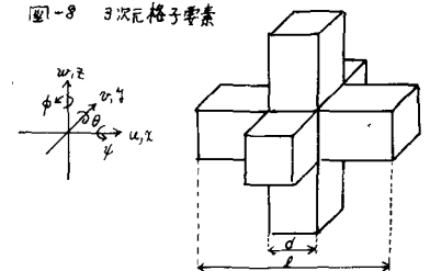
図-8 3次元格子要素
