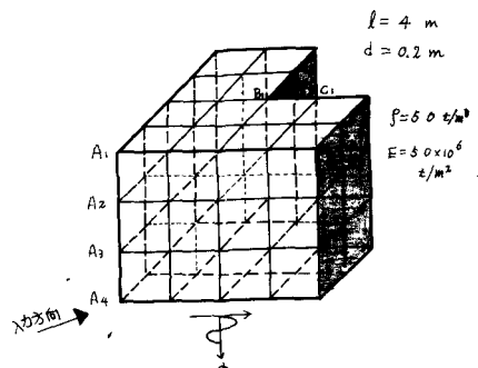
図-9 3次元骨組構造物
