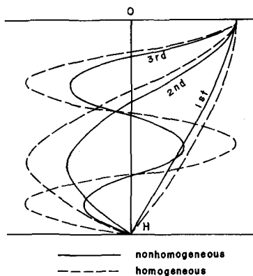
図-2 固有関数
