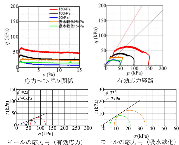
図 5 試験結果 (締固め度 90%・中型供試体)
