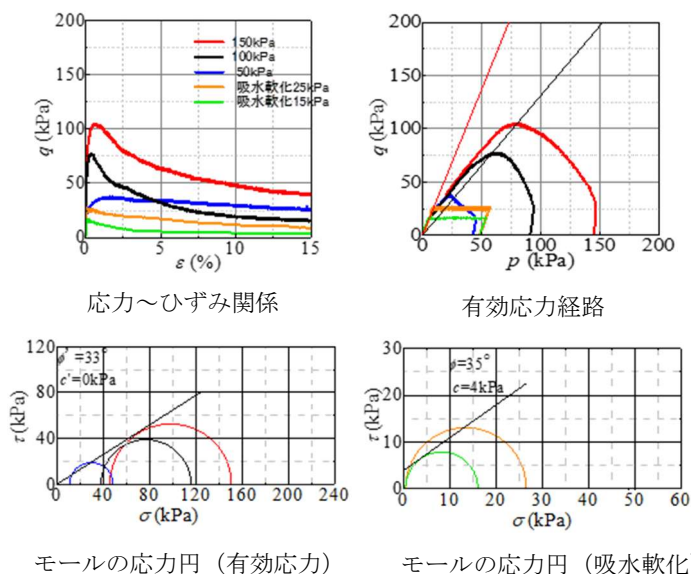
図2 試験結果（締固め度95%・大型供試体）
