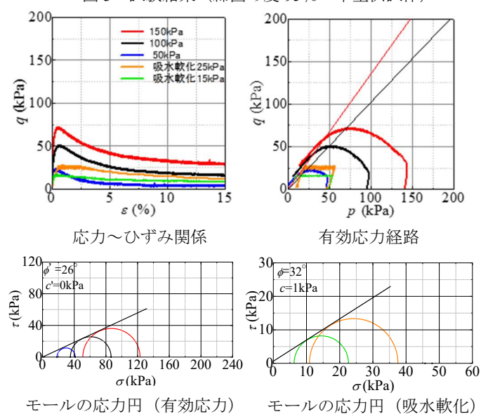
図 4 試験結果 (締固め度 90%・大型供試体)
