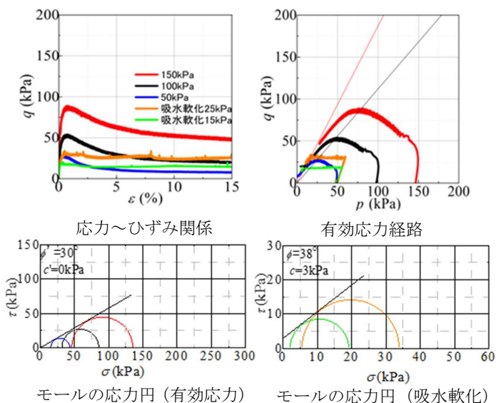
図 3 試験結果 (締固め度 95%・中型供試体)
