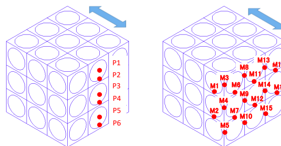
(a) 水圧計設置位置
