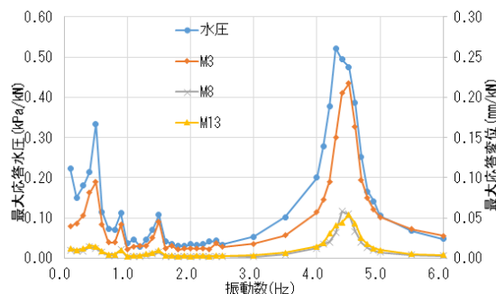
図-2 スweep試験 (H=2500mm) 水圧-開き量応答値
