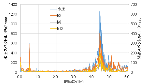
図-3 東北地方太平洋沖地震 (H=2500mm)
