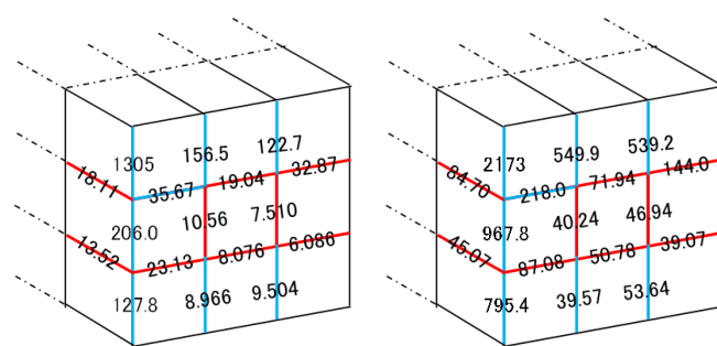
(a) 角度 0 度, 0.5Hz, 45mm (b) 角度 0 度, 4.5Hz, 1mm
