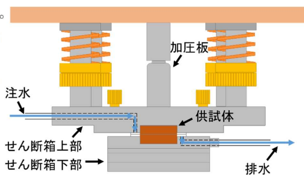
図1 一面せん断試験機模式図
