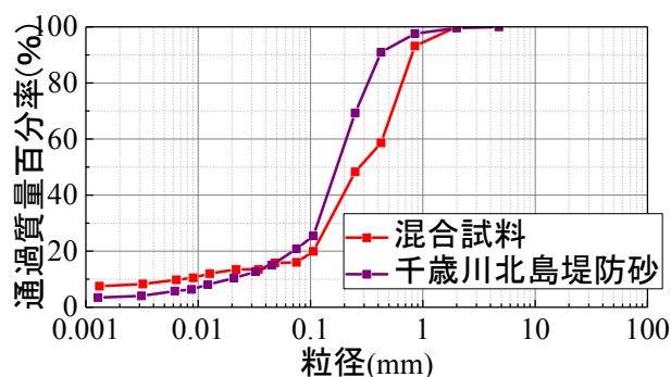
図2 試験試料と実堤防砂の粒度分布
