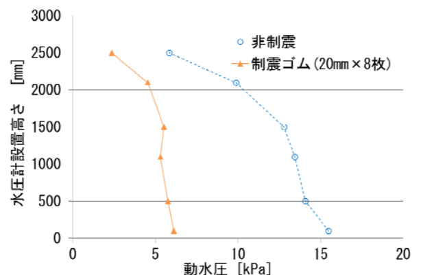
図-4 高さ方向の動水圧分布
