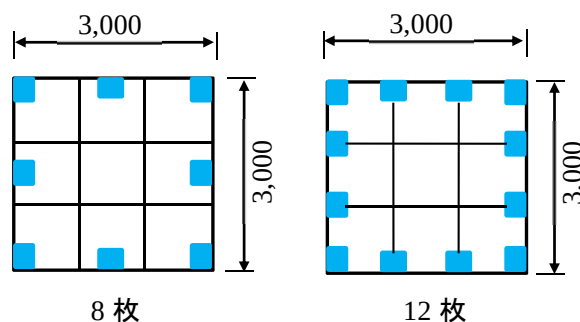
図-2 制震ゴム板の配置
