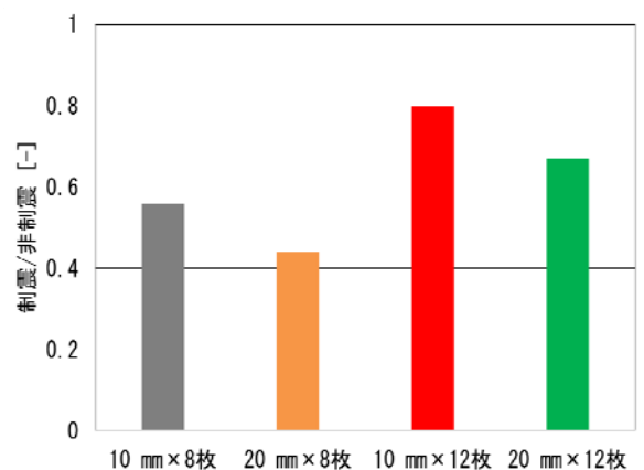
図-5 動水圧抑制効果
