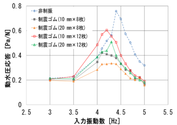
図-3 入力振動数に対する動水圧応答の変化
