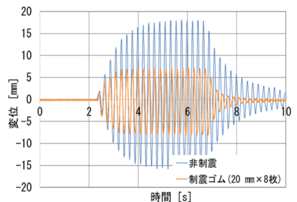
図-6 貯水槽の変位
