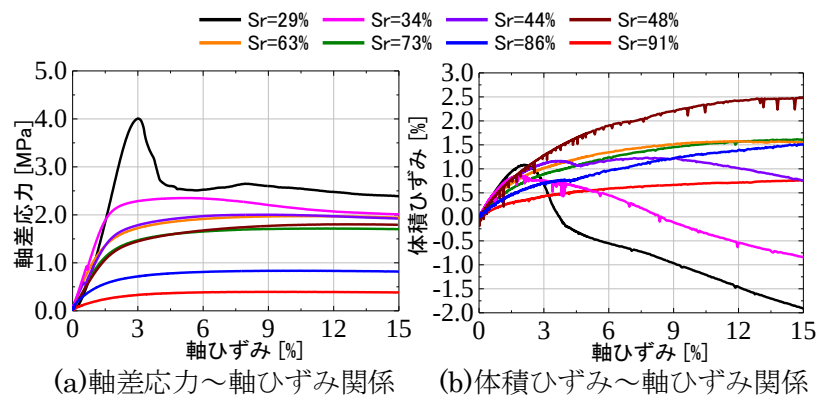
図3 各種不飽和供試体の非排気非排水三軸試験結果
