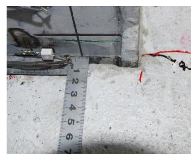
写真-1 根巻コンクリート 上部に発生した隙間
