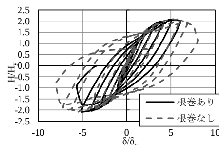
図-2 水平荷重-変位関係 (橋軸直角方向)
