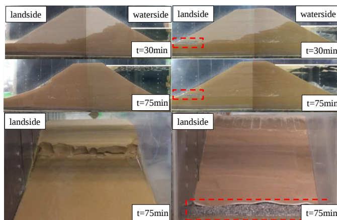
図-2 水位上昇時における堤体断面と法面の様子 左：無対策堤防，右：対策堤防 (ドレーン工)
