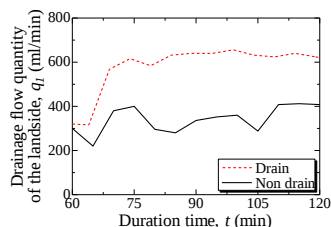
図-4 水位上昇時における堤内側排水流量
