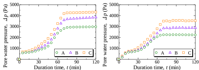
図-3 水位上昇時における間隙水圧の経時変化 左：無対策堤防，右：対策堤防（ドレーン工）
