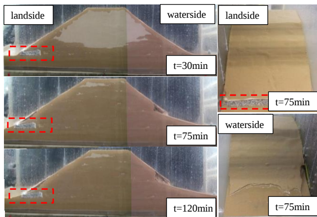
図-5 降雨時における堤体断面と法面の様子 右上：堤内側，右下：堤外側
