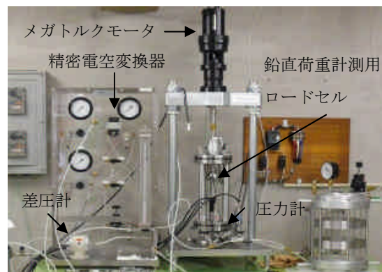
図 1 高圧三軸試験装置
