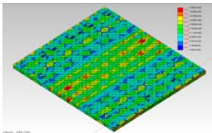
図 - 4 応力度コンター図
