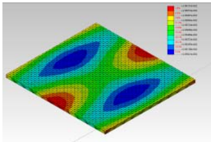
図 - 3 鉛直変位コンター図
