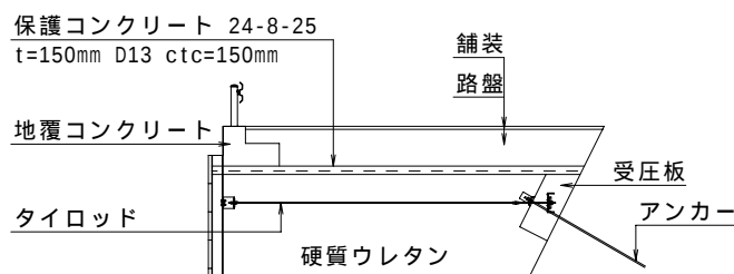
図 - 1 硬質ウレタン上部標準構造図
