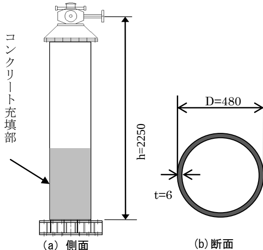
図-1 実験供試体図 (mm)
