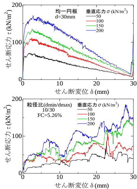
図 1 せん断変位とせん断応力の関係
