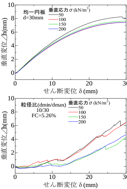
図 2 せん断変位と垂直変位の関係
