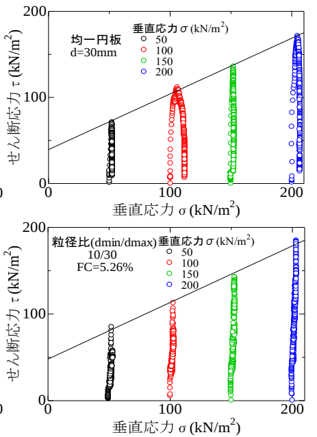
図 3 垂直応力とせん断応力の関係
