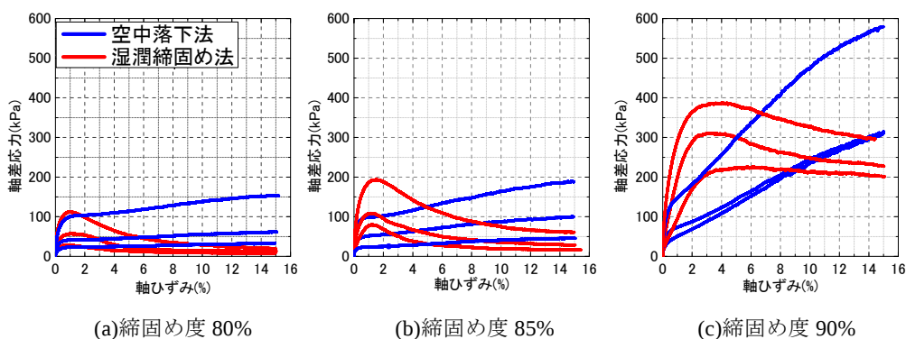
図2 応力～ひずみ関係
