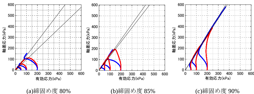
図3 有効応力経路
