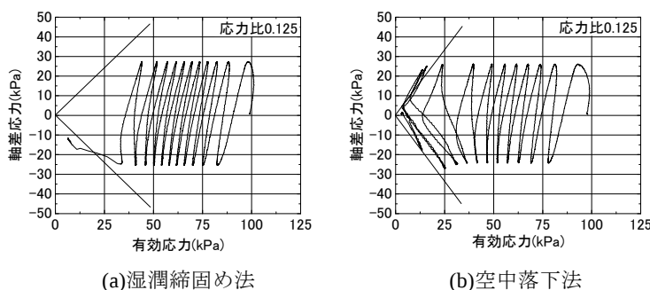
図 5 有効応力経路
