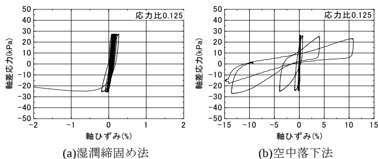
図 4 応力～ひずみ関係
