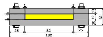
図-5 拘束材断面図
