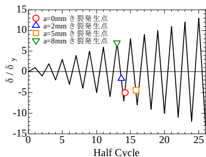
図-2 き裂発生点の比較
