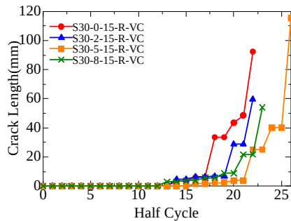
図-3 き裂進展の比較
