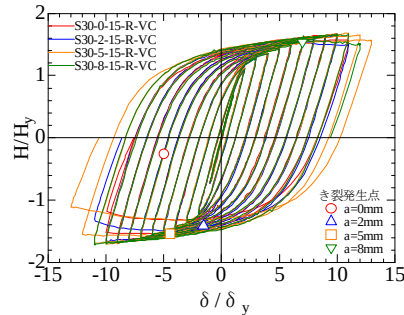
図-4 荷重－変位履歴曲線
