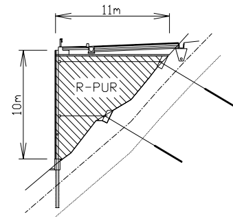
図 4 断面-2
