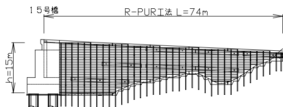
図 2 正面展開図
