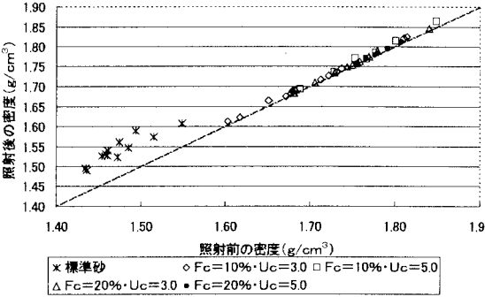
図-5 照射前と照射後の密度関係
