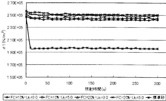
図-3 主応力差と除荷時間
