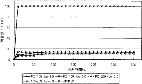
図-4 条件別荷重低下率
