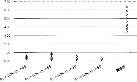
図-6 条件別密度増加率
